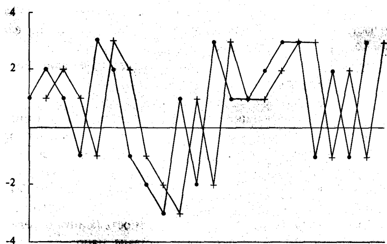
Рисунок 1-5 Отдельные результаты 21 сделки, сдвинутые на 1 сделку
