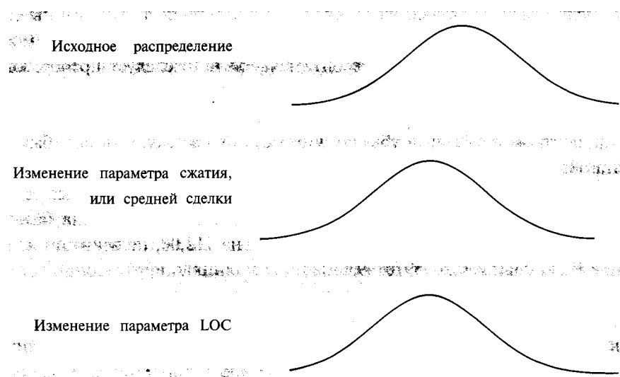
Рисунок 4-12 Изменение параметра расположения распределения
