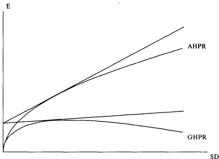
Рисунок 7-5 АНПР, ГНПР и их линии CML
